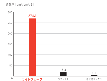
通気性比較
