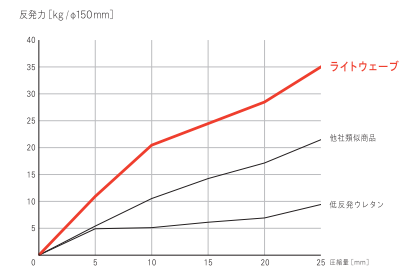
反発力比較
